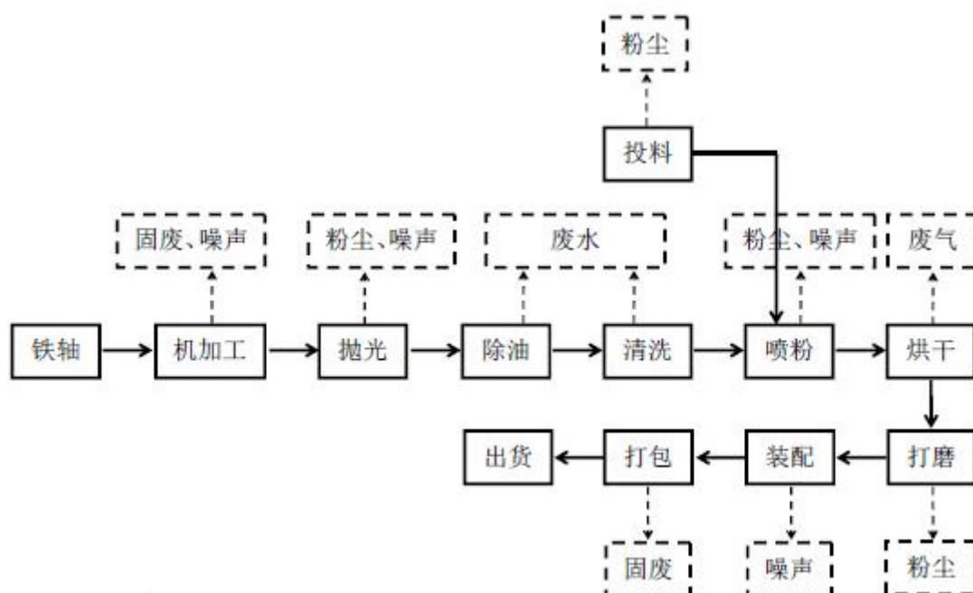
图2-1 项目生产流程图
