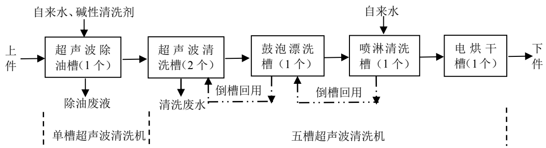
图 2-1 除油清洗线工作示意图
