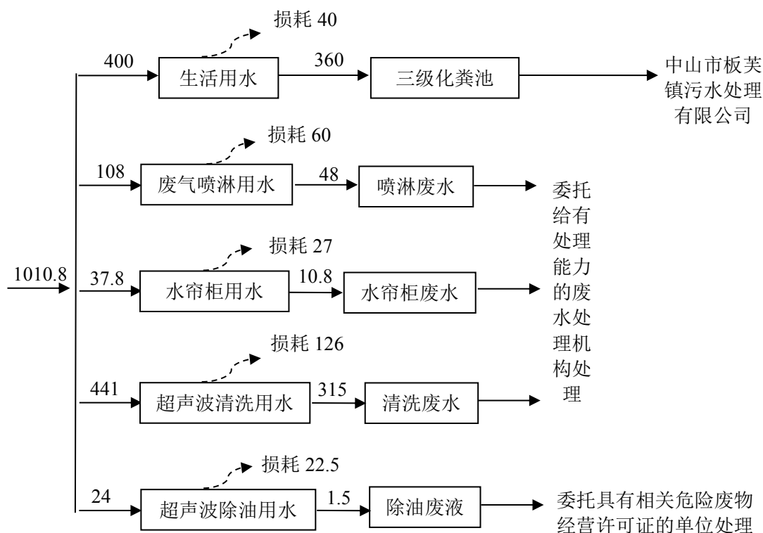
图 2-2 项目水平衡图（单位：t/a）
