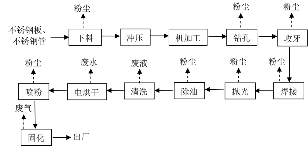
图 2-4 展示五金工艺流程图
