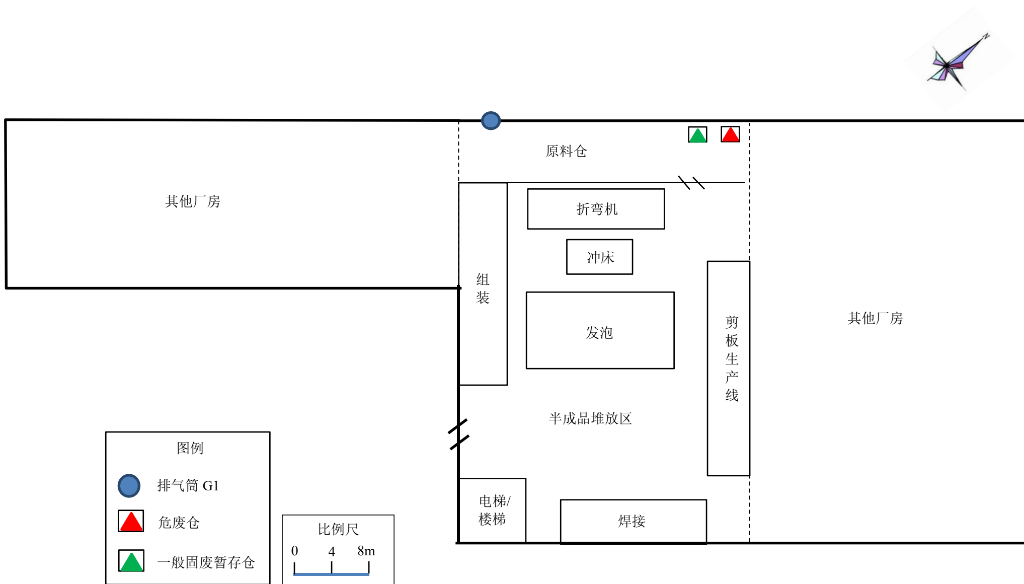
附图 3-1 一层车间平面布置图
