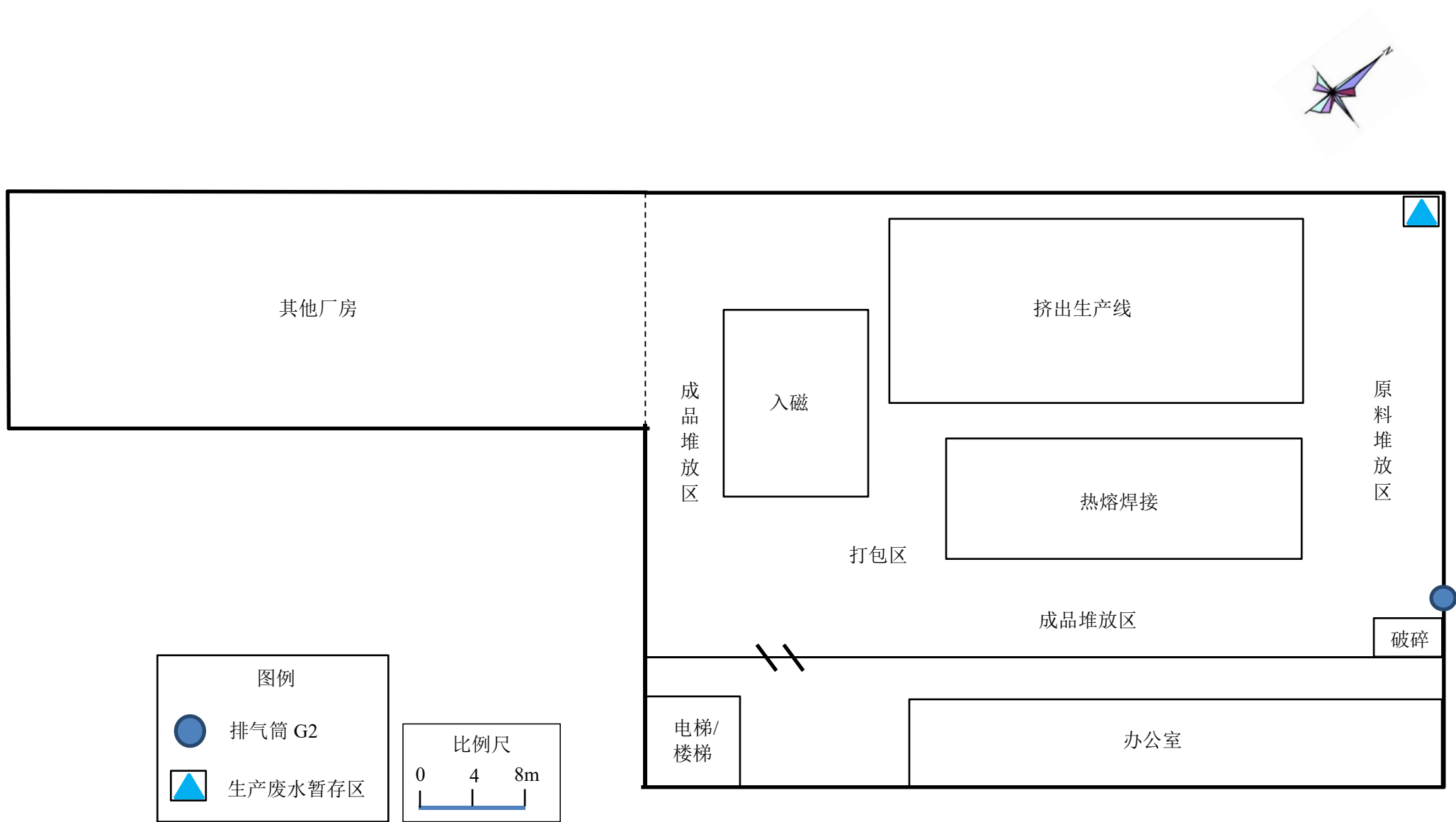
附图 3-2 二层车间平面布置图
