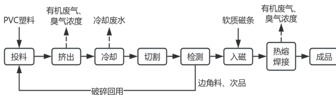
图 3 门封条生产工艺流程图
