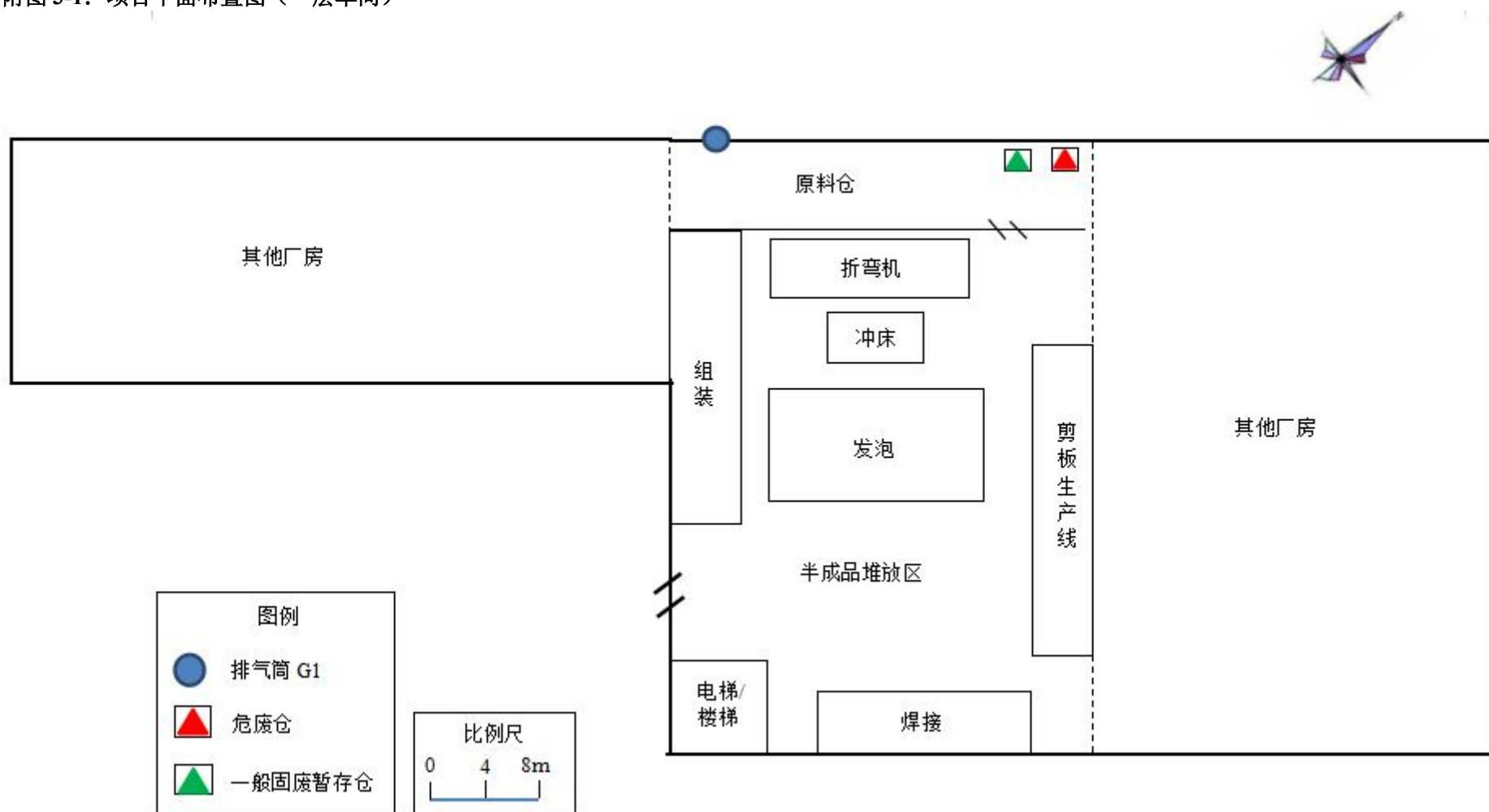
附图 3-1：项目平面布置图（一层车间）
