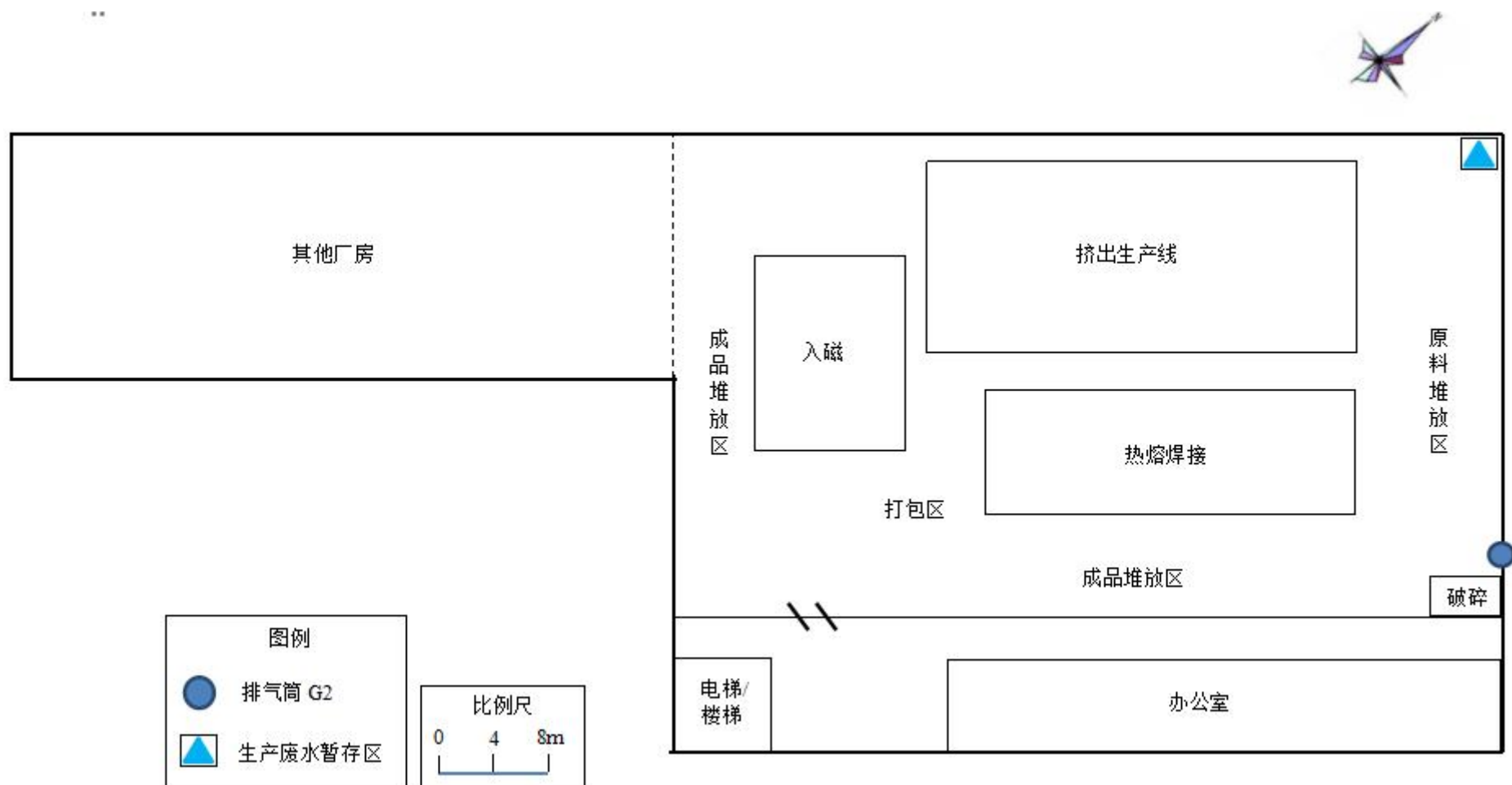
附图 3-2：项目平面布置图（二层车间）
