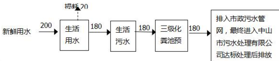
图 2-1 项目实际水平衡图（单位：t/a）
