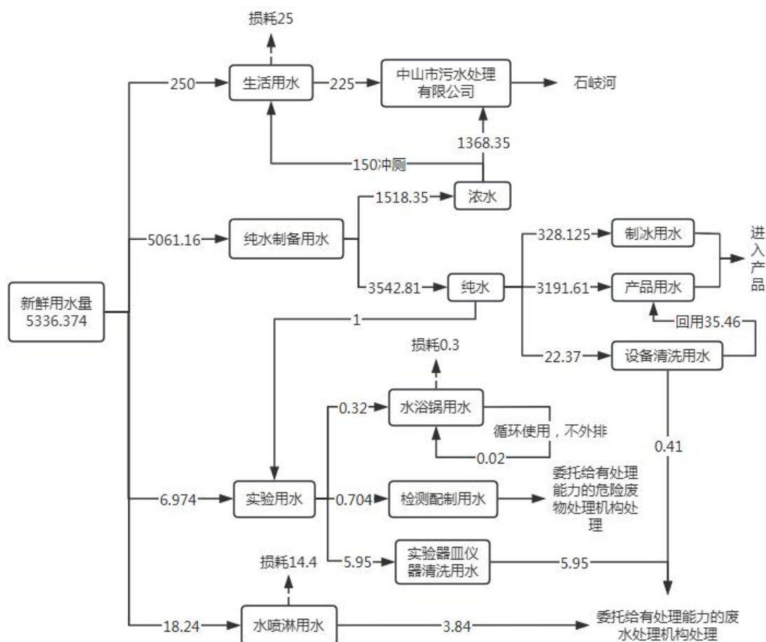
图 2-1 项目实际水平衡图（单位：t/a）
