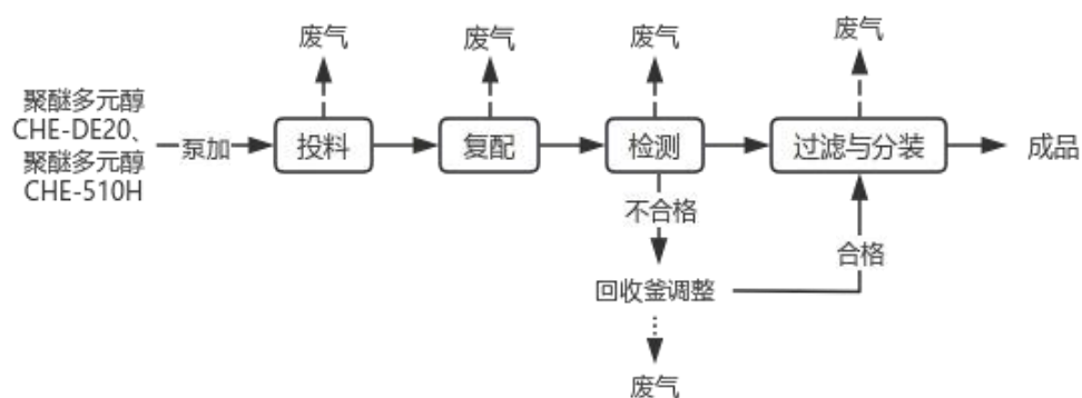
图2-4 聚醚消泡剂生产工艺流程图
