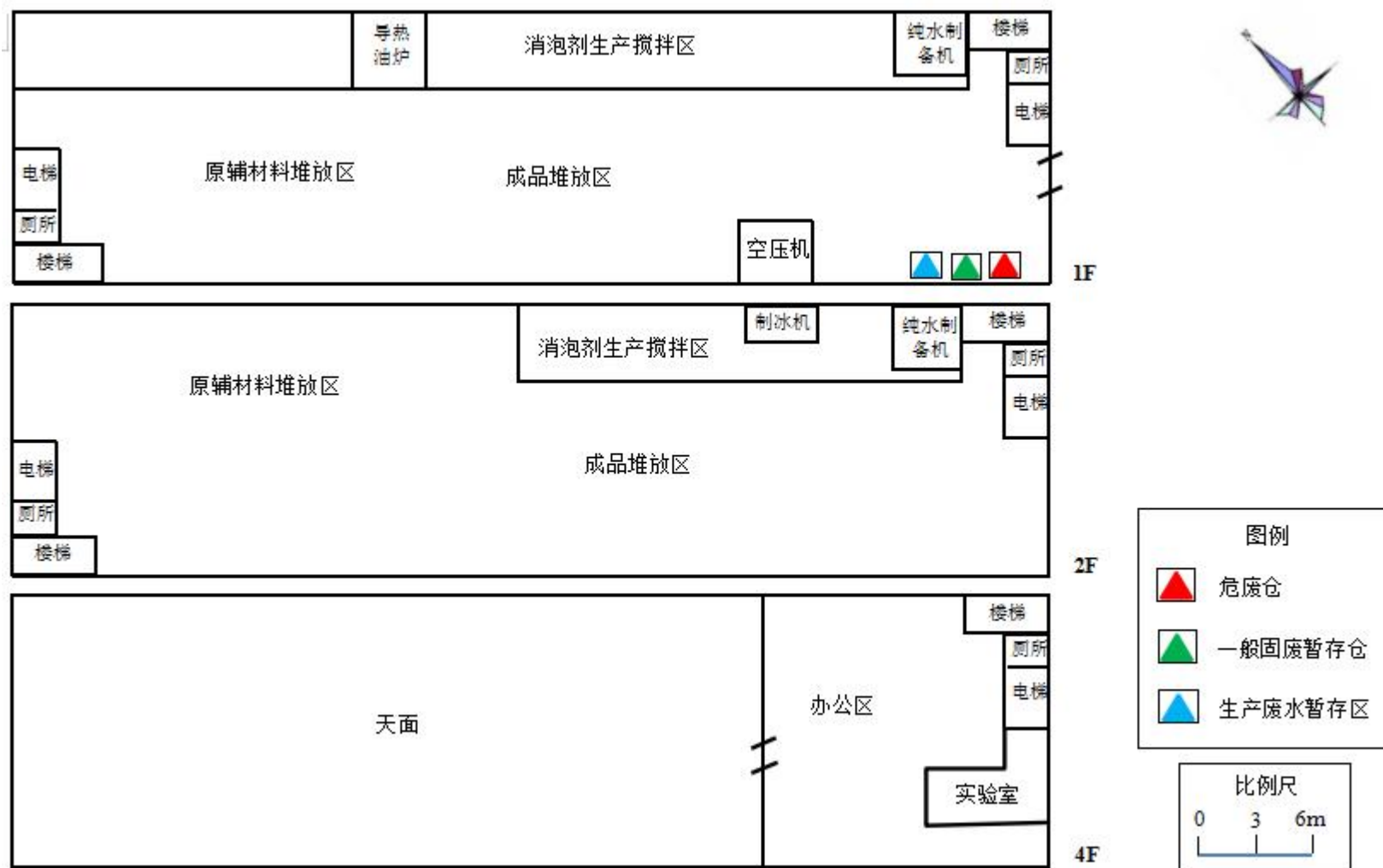
附图 3-2：项目平面布置
