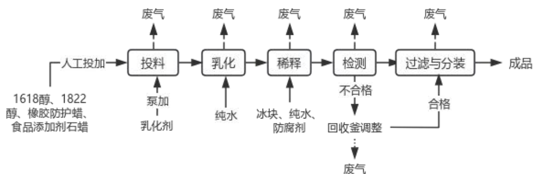
图2-3 高碳醇消泡剂生产工艺流程图
