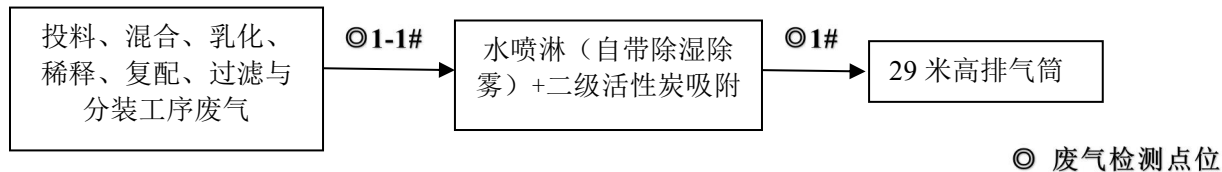
图 3-1 废气处理工艺流程图
