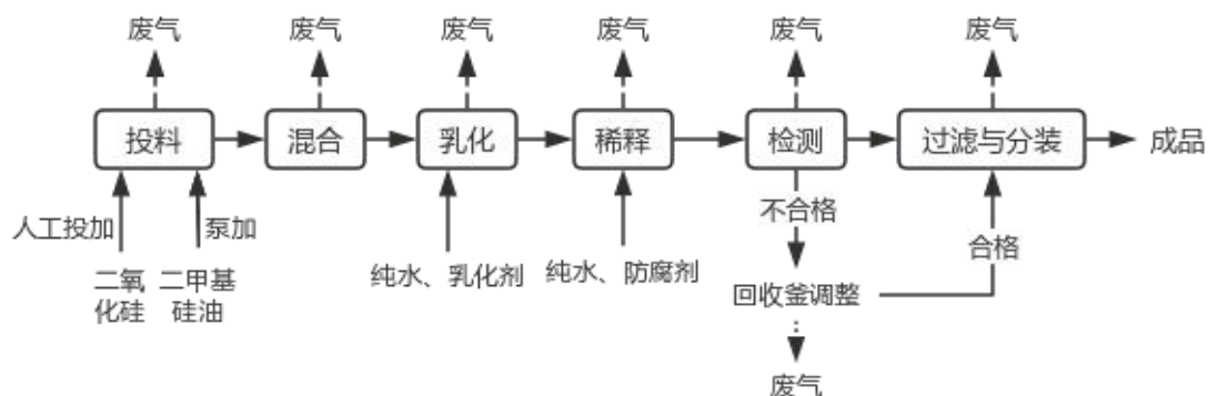
图2-2 有机硅消泡剂生产工艺流程图
